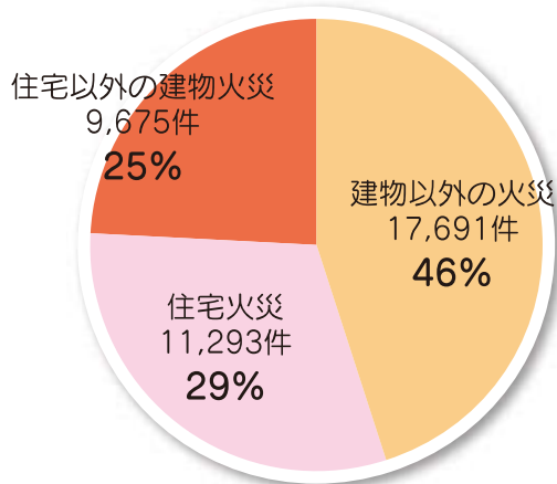
令和5年中の火災件数
