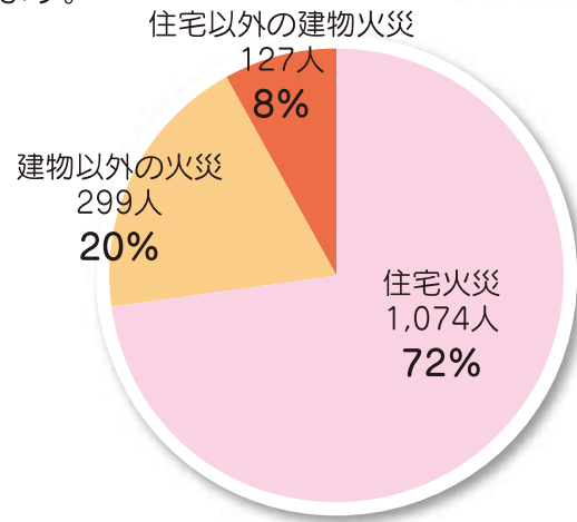
令和5年中の火災死者数
