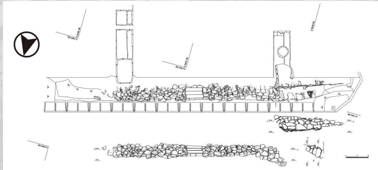
隠居曲輪で見つかった石垣の平面図・立面図
