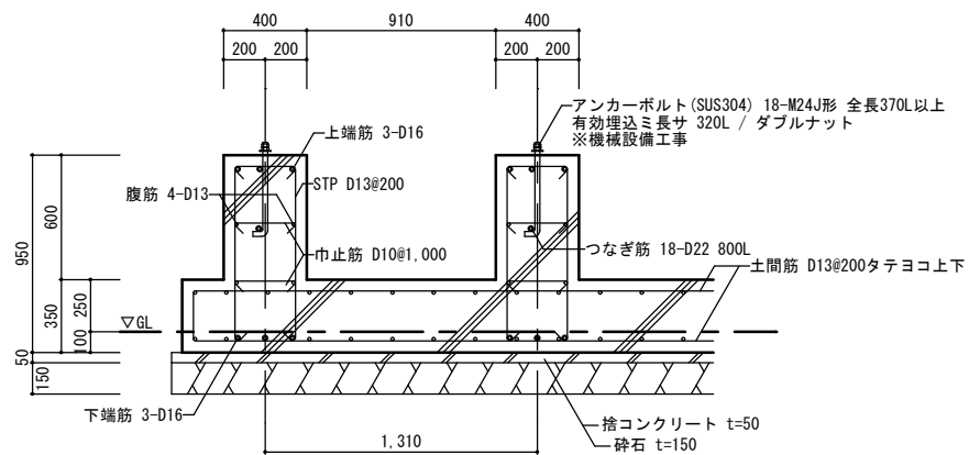
基礎詳細図 1/20
