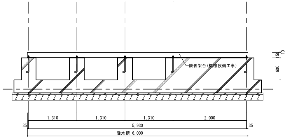
本体立面図 1/30
