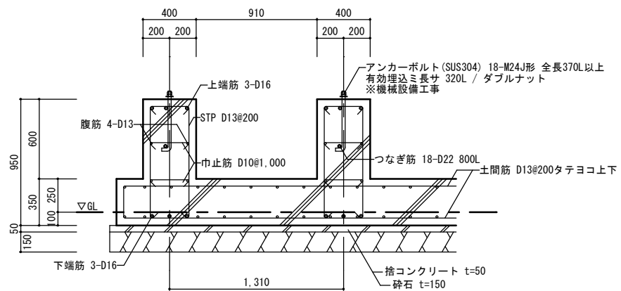
基礎詳細図 1/20
