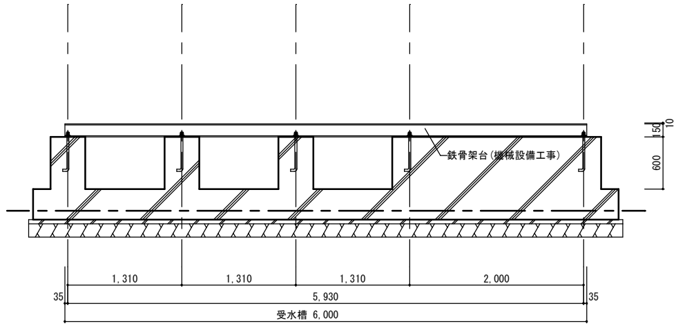
本体立面図 1/30
