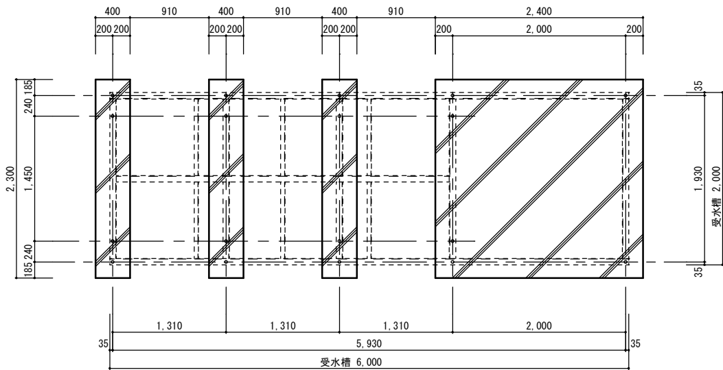
受台伏図 1/30
