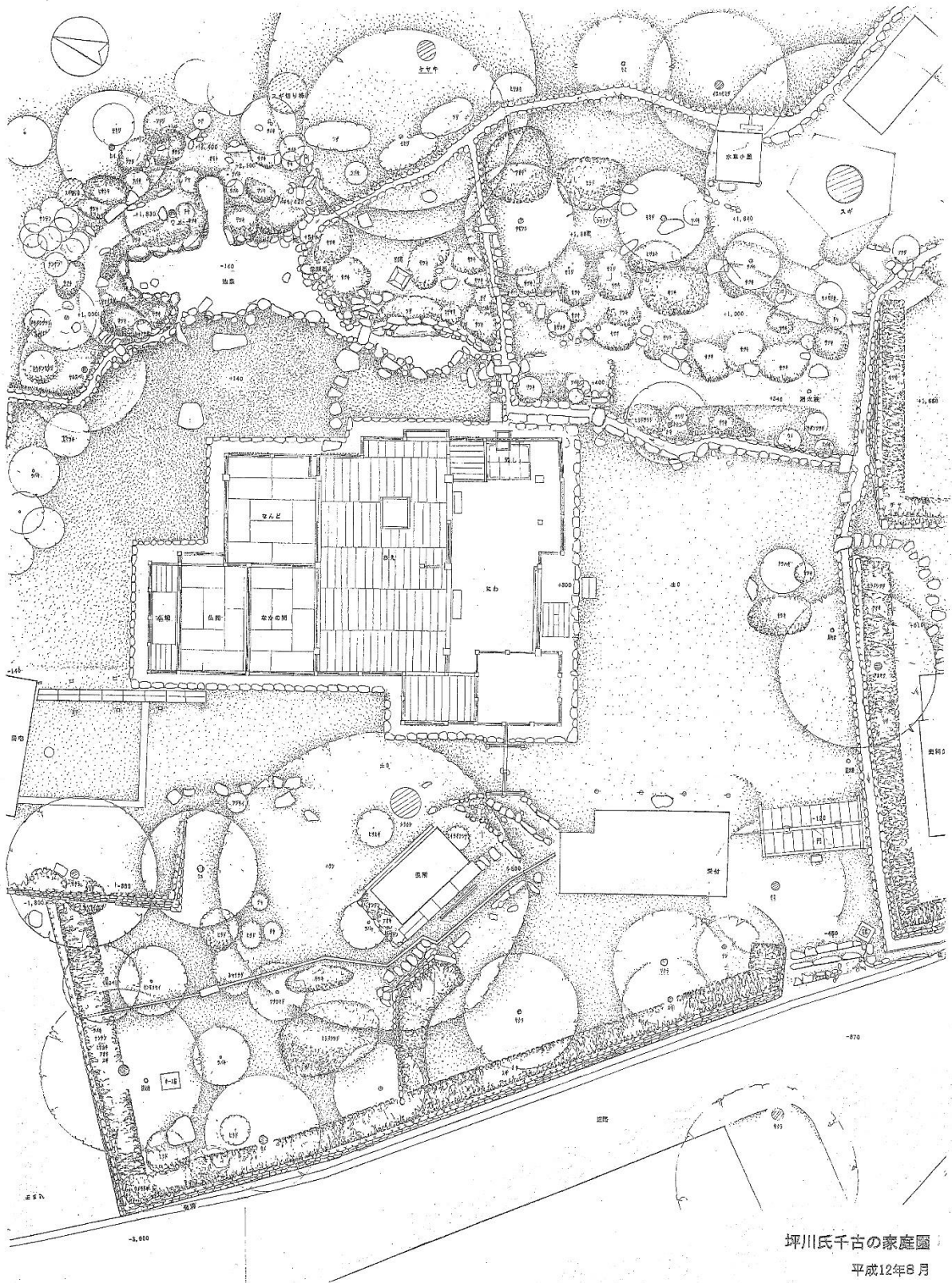
坪川家庭園平面図（平成12年8月）（作図：齋藤忠一氏）
