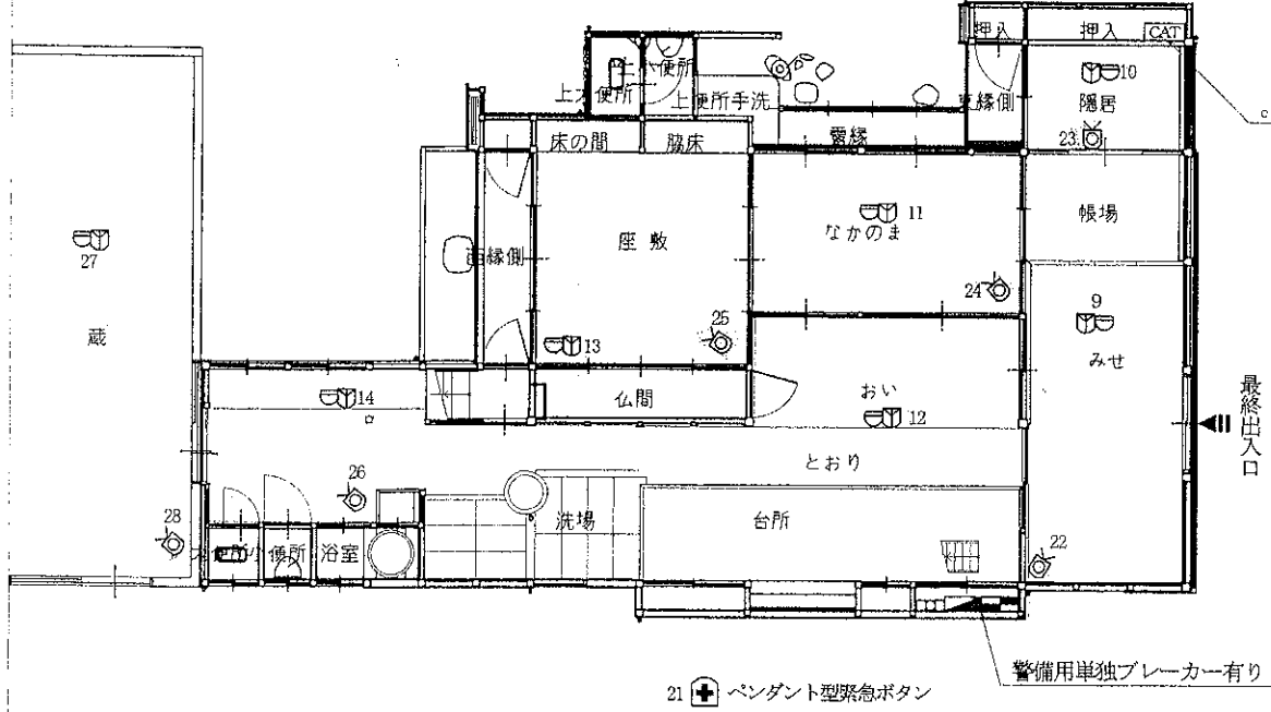
1階平面図
