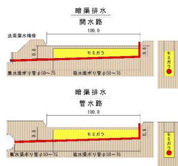
標準断面図
