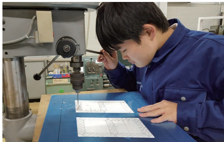
▲LEDをはめ込む基盤に穴をあけています
