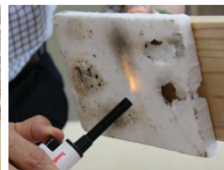
▲不燃化を施した素材は、燃焼させても炎が上らず有害な煙やガスも発生しない(写真は発泡スチロール)
