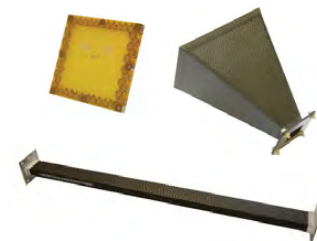
▲当社が設計・開発したはやぶさのアンテナと導波管(同型)。三軸織物技術を応用することで、従来よりも6分の1の軽さを実現
