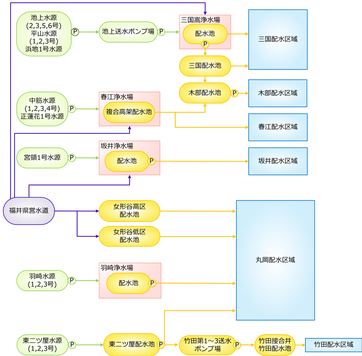
図 2-2 配水フロー
