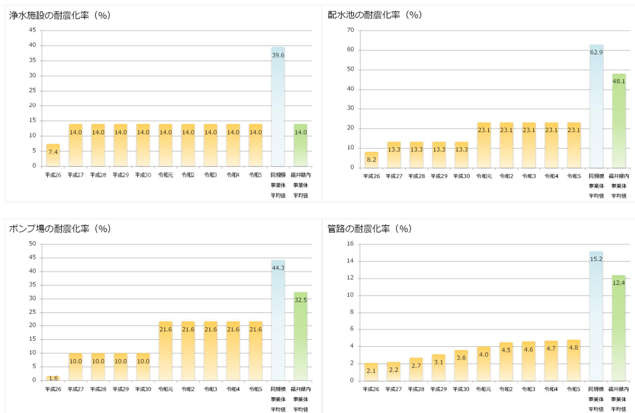
図 2-5 耐震化率 (左上：浄水施設、右上：配水池、左下：ポンプ場、右下：管路)
